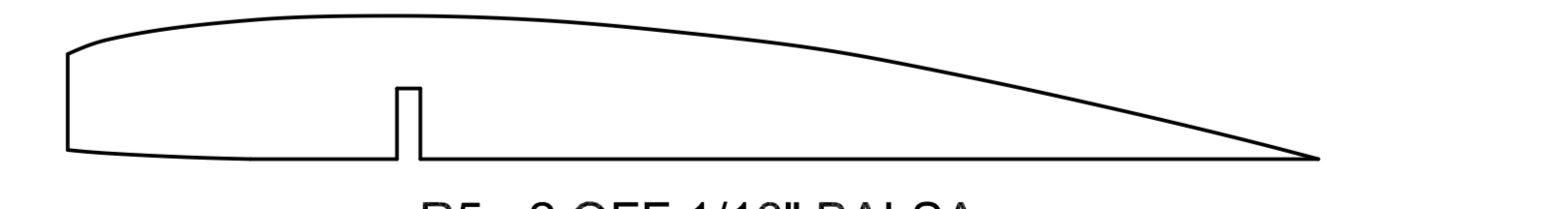
R5 - 2 OFF 1/16" Balsa
